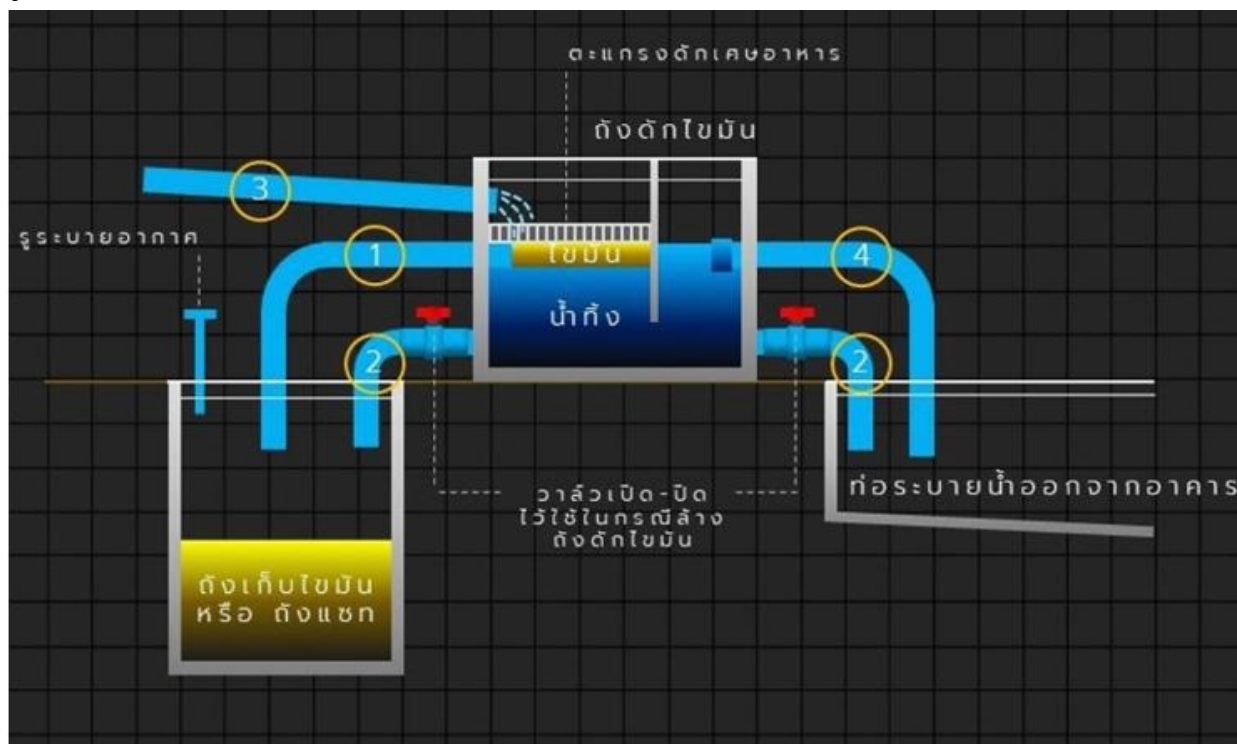
ระบบดักจับไขมัน (Grease Trap) และบ่อเกรอะ (Septic Tank)
